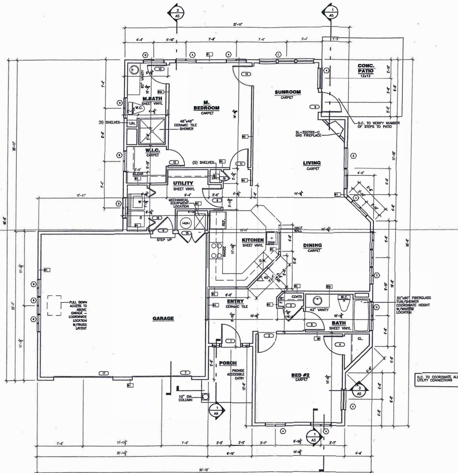
SCALE: 1/4"=1'-0"
